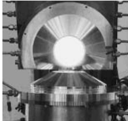
Die Öffnung des Solarreaktors nach einem Experiment
